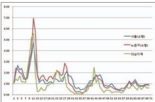
그림 4. 거래량 분포
