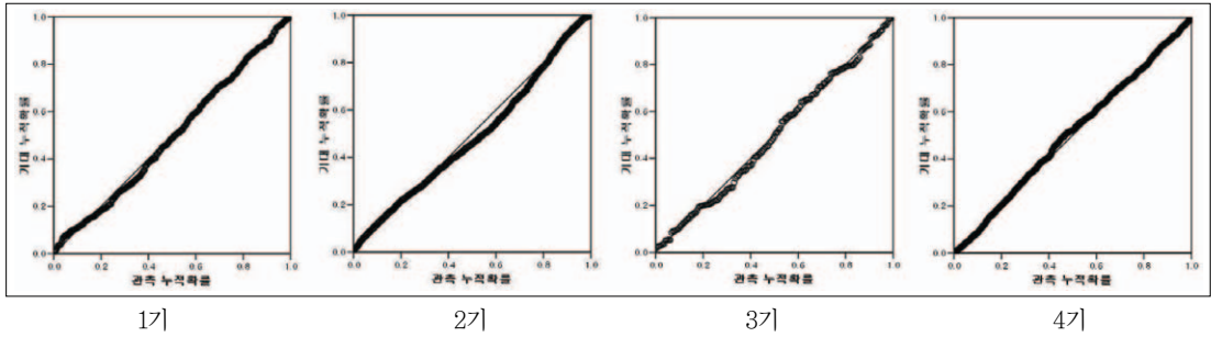
그림 6. 기간별 정규확률도
